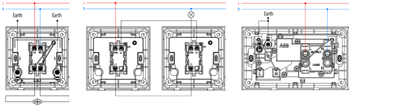
1G 1W DP switch
