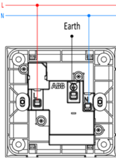
1G universal switch socket
